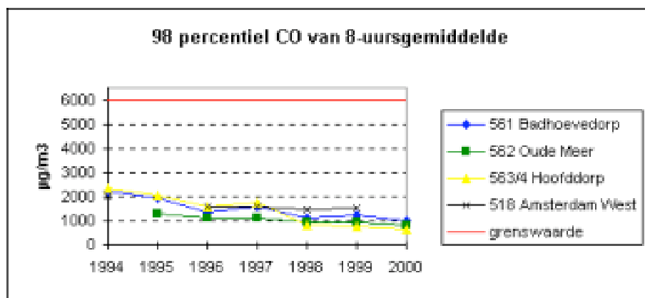
Figuur 5.2: Ontwikkeling koolmonoxide
